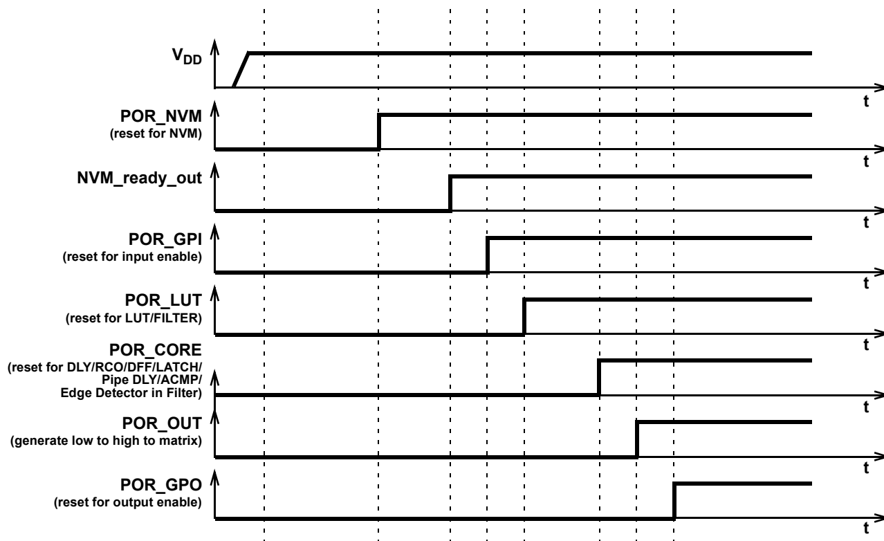
Figure 145: POR Sequence
