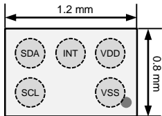
<WLCSP, Top view>
